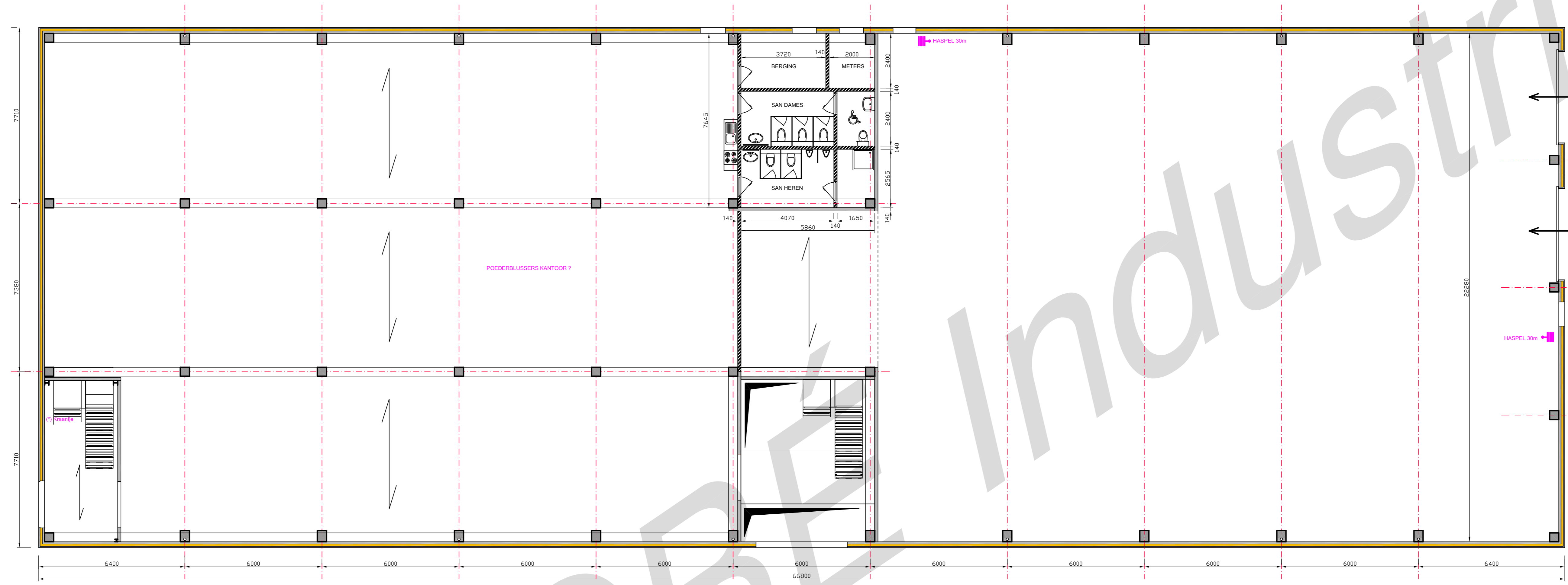
GRONDPLAN
